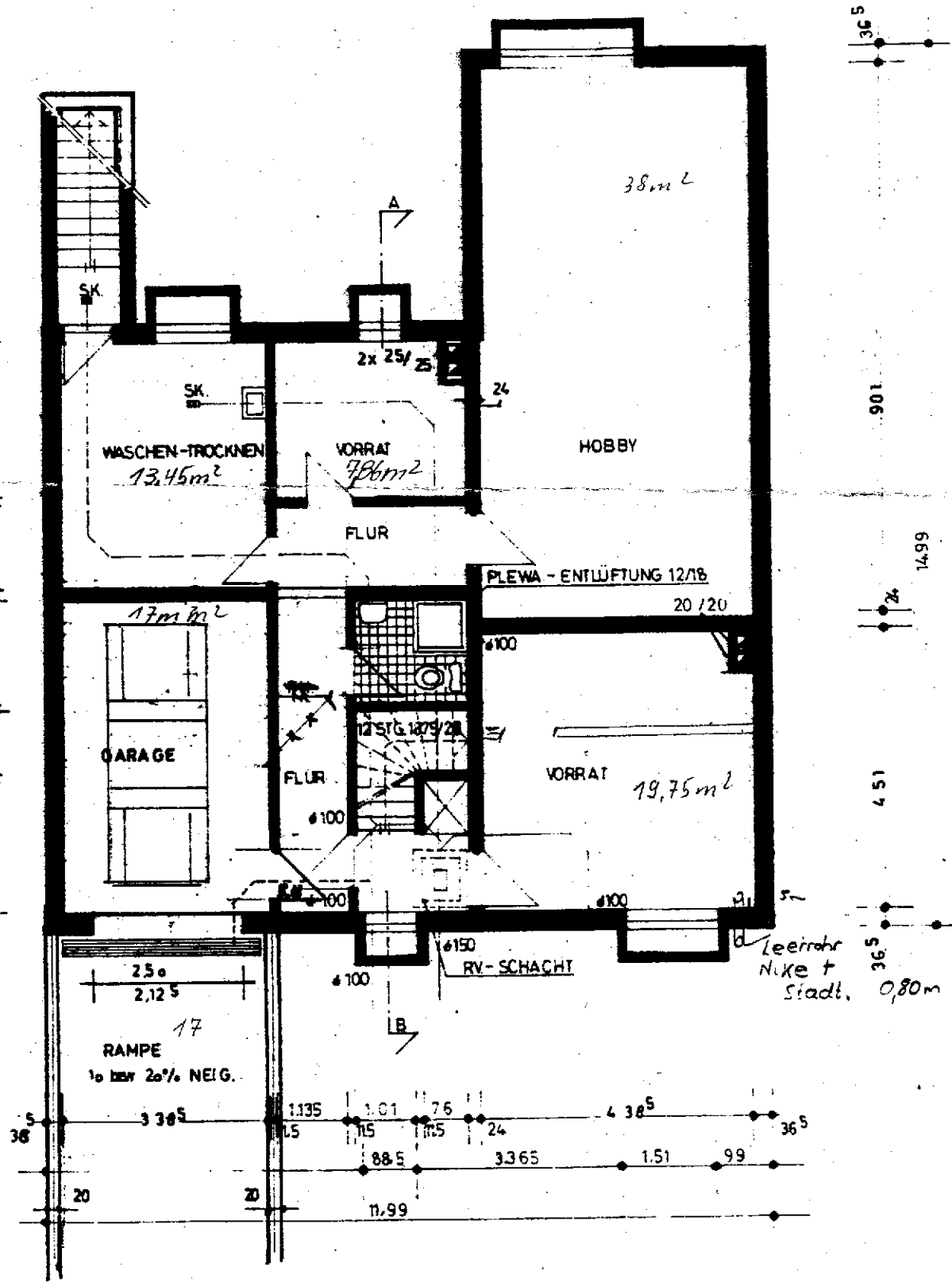
KELLERGESCHOSS
