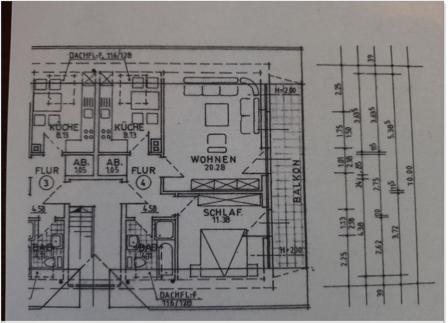
Grundriss
